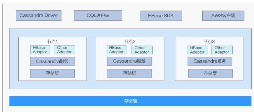
图 1-1 GeminiDB HBase 接口架构图
